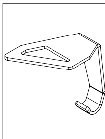
SUPPORT, CROCHET EN T DROIT U725 BIKINI Qté. 1
